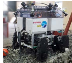
当社が共同開発したクローラーロボット（©海洋研究開発機構）
